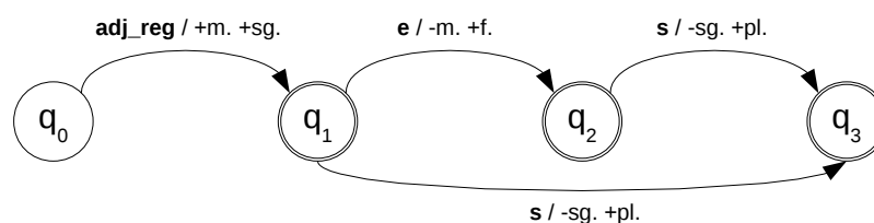
Figure 1.6 Exemple d'automate à états finis étiquetant en genre et en nombre un adjectif régulier en français
